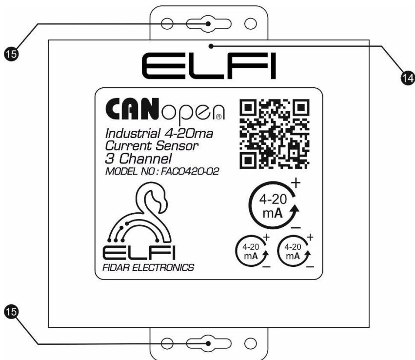
شکل ۳: نمای روبه روی Node جریان ۴-۲۰ میلی آمپر سه کانال
