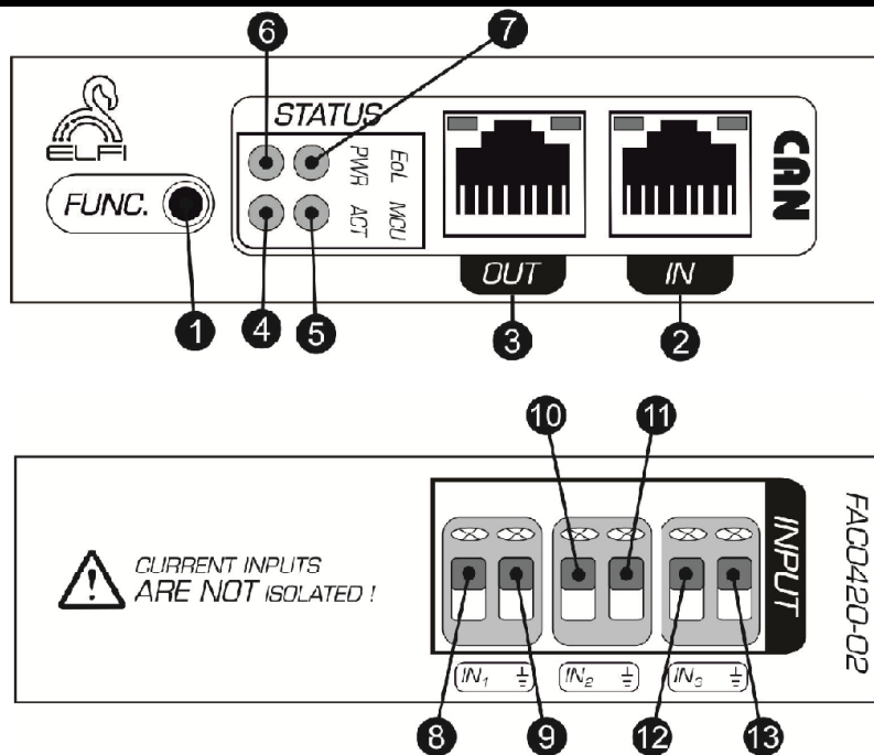
شکل ۲: نمای جانبی Node جریان ۴-۲۰ میلی آمپر سه کانال
