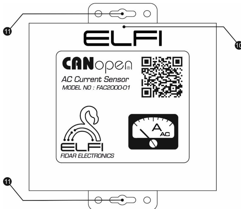
شکل ۳: نمای روبه روی Node جریان متناوب (AC)
