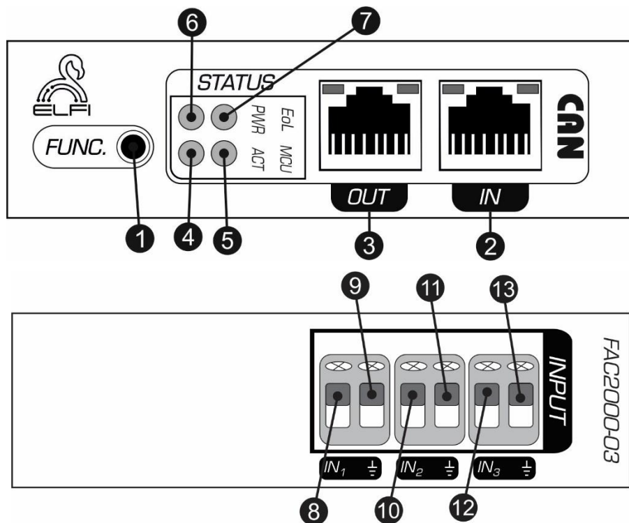
شکل ۲: نمای جانبی Node جریان متناوب (AC)
