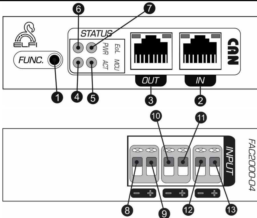
شکل ۲: نمای جانبی Node جریان DC
