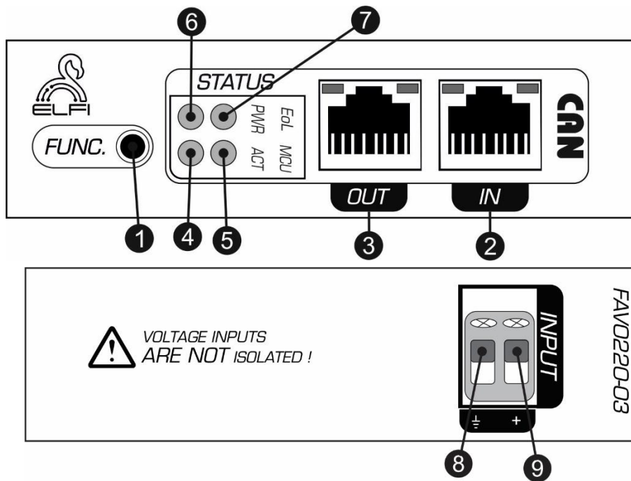
شکل ۲: نمای جانبی Node سطح ولتاژ متناوب
