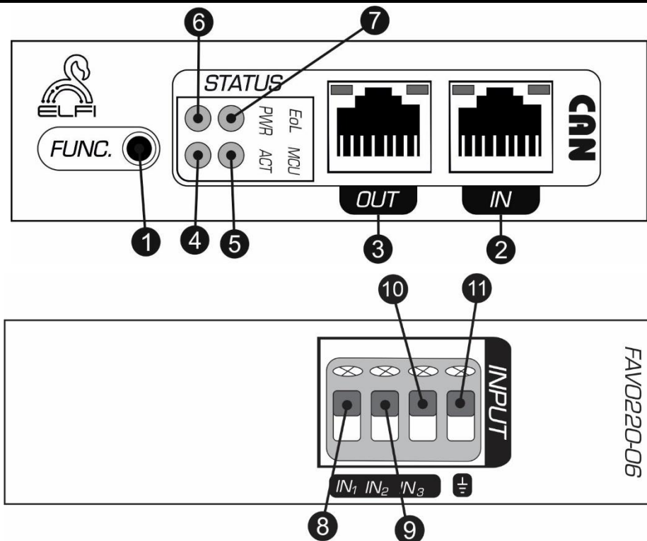
شکل ۲: نمای جانبی Node دتکتور ولتاژ مستقیم سه کانال
