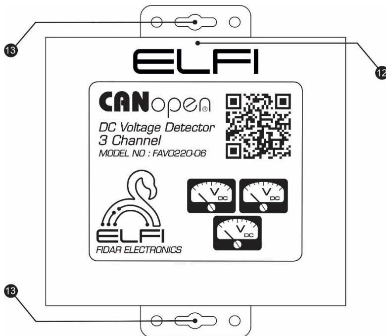
شکل ۳: نمای روبه روی Node دتکتور ولتاژ مستقیم سه کانال
