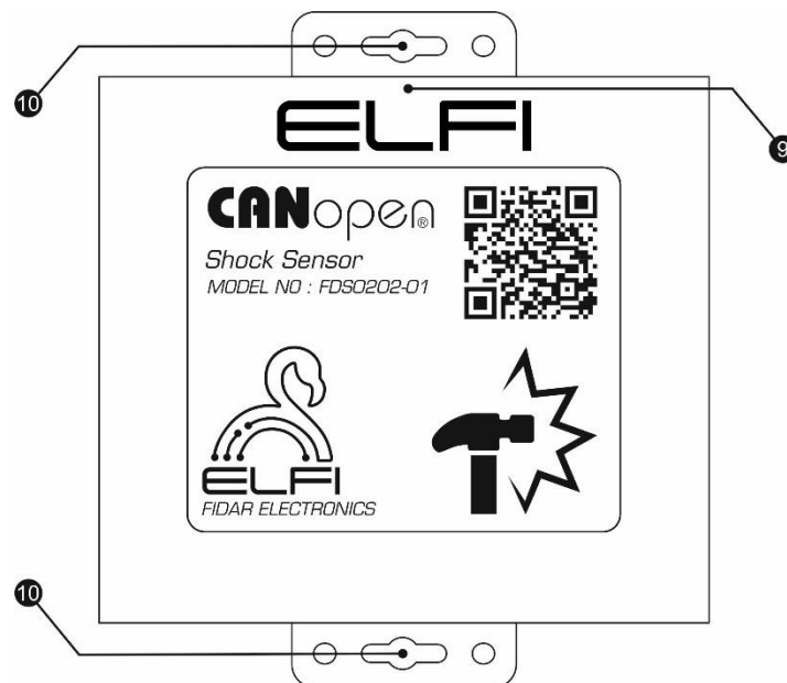
شکل ۳: نمای روبه روی Node تشخیص ضربه
