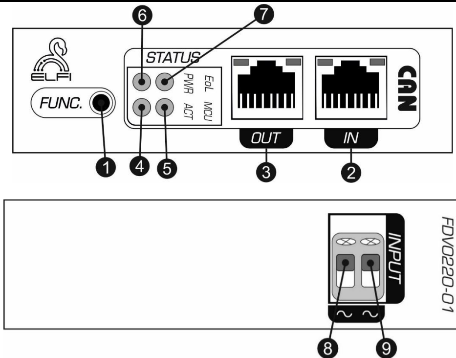
شکل ۲: نمای جانبی Node دتکتور ولتاژ متناوب تک کانال
