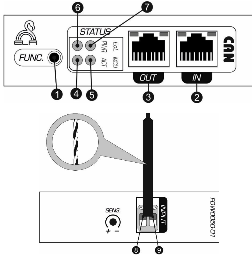
شکل ۲: نمای جانبی Node تشخیص نشتی آب
