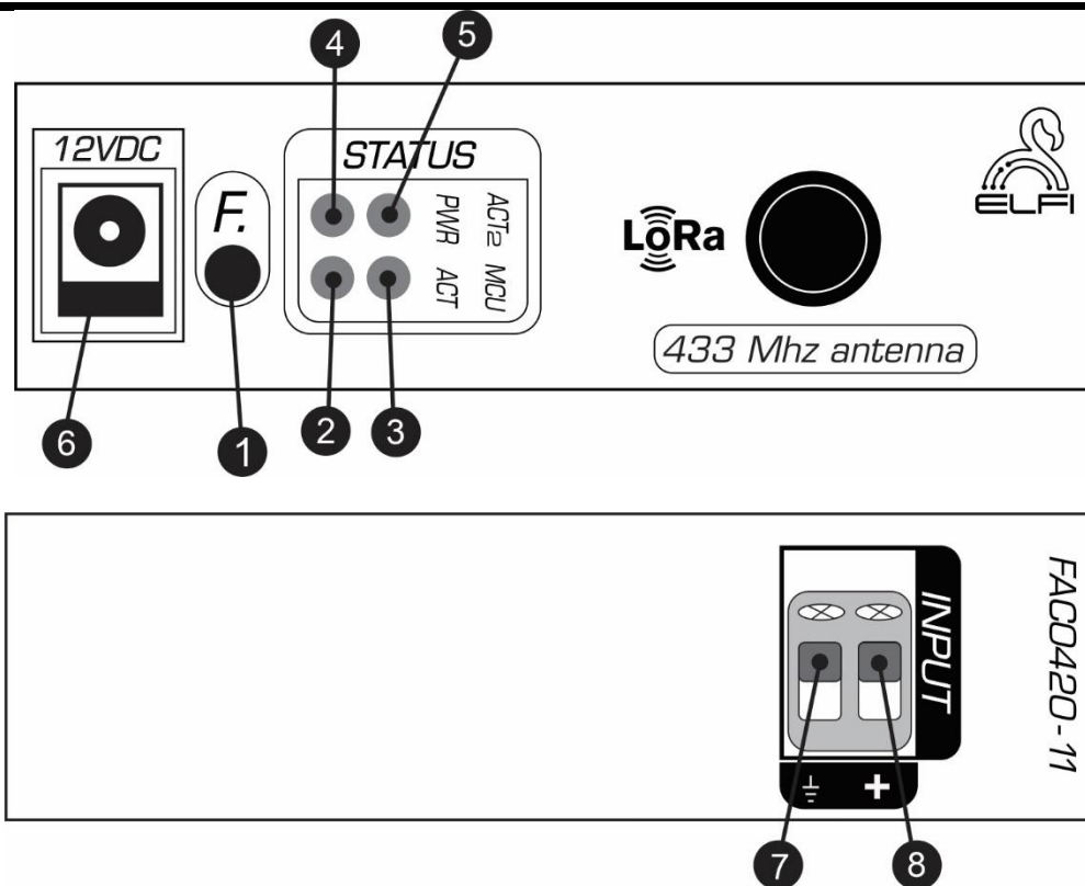
شکل ۲: نمای جانبی Node ۲۰-۴ میلی آمپر تک کانال بی سیم
