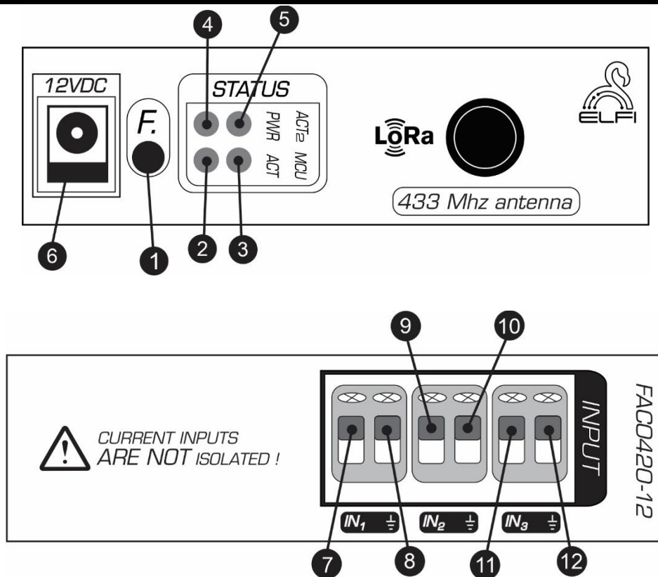
شکل ۲: نمای جانبی Node جریان ۲۰-۴ میلی آمپر سه کانال بی سیم
