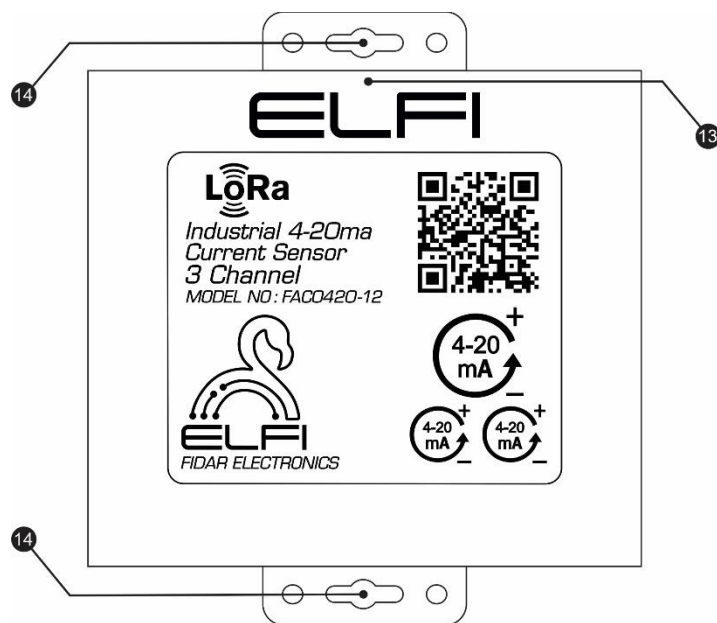
شکل ۳: نمای روبه روی Node جریان ۲۰-۴ میلی آمپر سه کانال بی سیم
