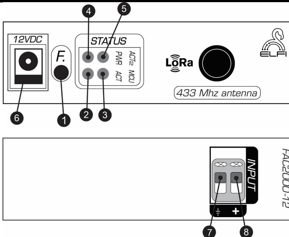
شکل ۲: نمای جانبی Node جریان DC تک کانال بی سیم
