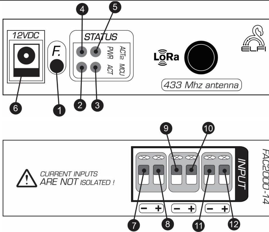
شکل ۲: نمای جانبی Node جریان DC سه کانال بی سیم
