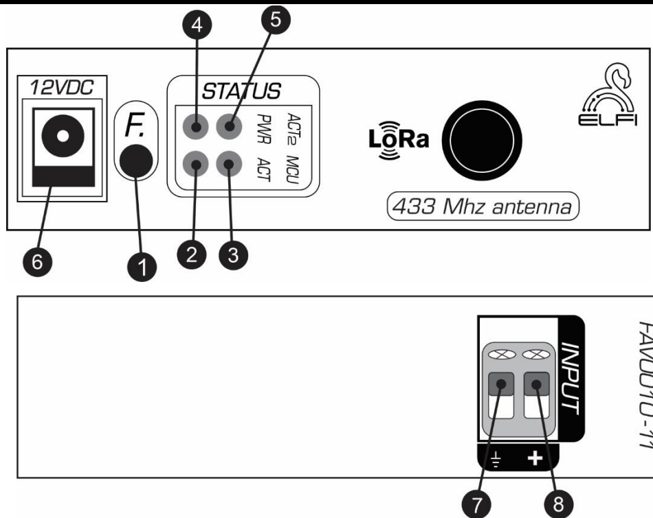
شکل ۲: نمای جانبی Node ° تا ° ۱ ولت مستقیم تک کانال بی سیم
