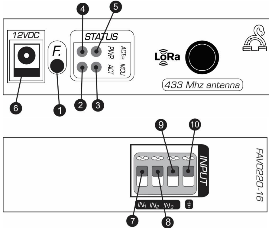
شکل ۲: نمای جانبی Node دتکتور ولتاژ مستقیم سه کانال بی سیم
