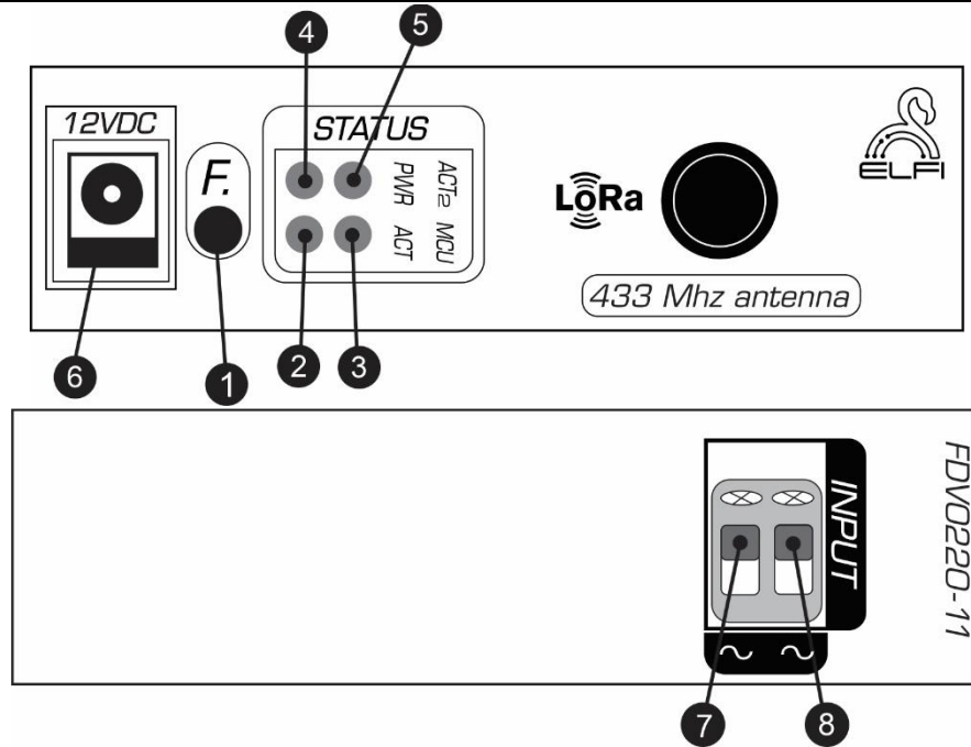
شکل ۲: نمای جانبی Node دتکتور ولتاژ متناوب تک کانال بی سیم
