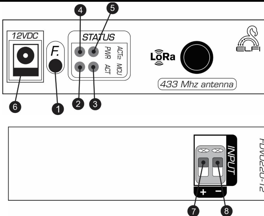
شکل ۲: نمای جانبی Node دتکتور ولتاژ مستقیم تک کانال بی سیم
