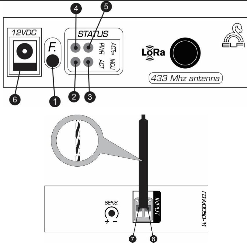
شکل ۲: نمای جانبی Node تشخیص نشتی آب بی سیم
