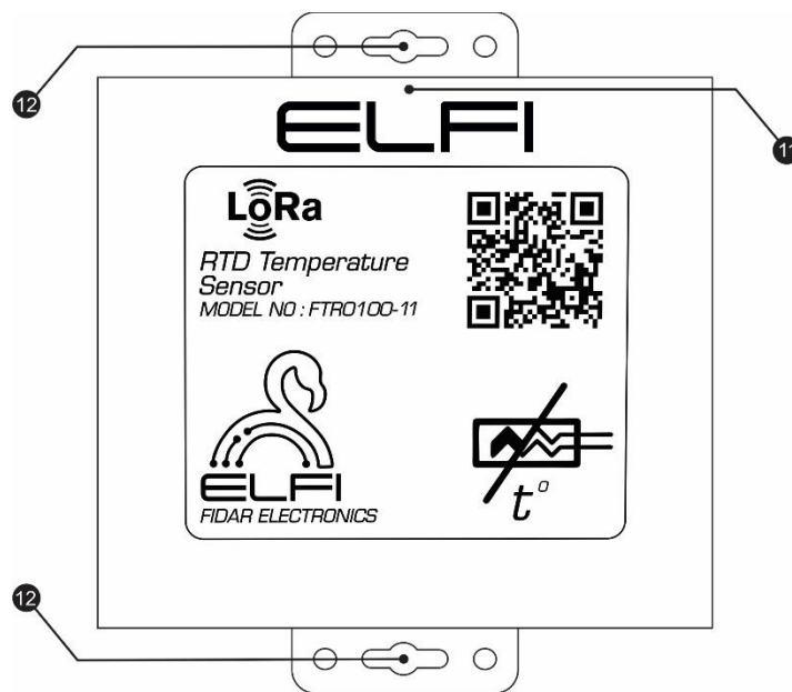
شکل ۳: نمای روبه روی Node دمای PT100 بی سیم
