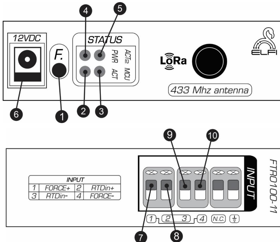
شکل ۲: نمای جانبی Node دمای PT100 بی سیم
