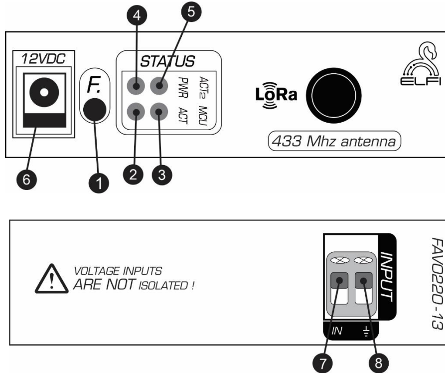
شکل ۲: نمای جانبی Node سطح ولتاژ متناوب بی سیم
