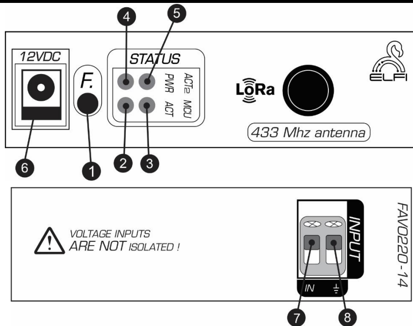
شکل ۲: نمای جانبی Node سطح ولتاژ مستقیم بی سیم
