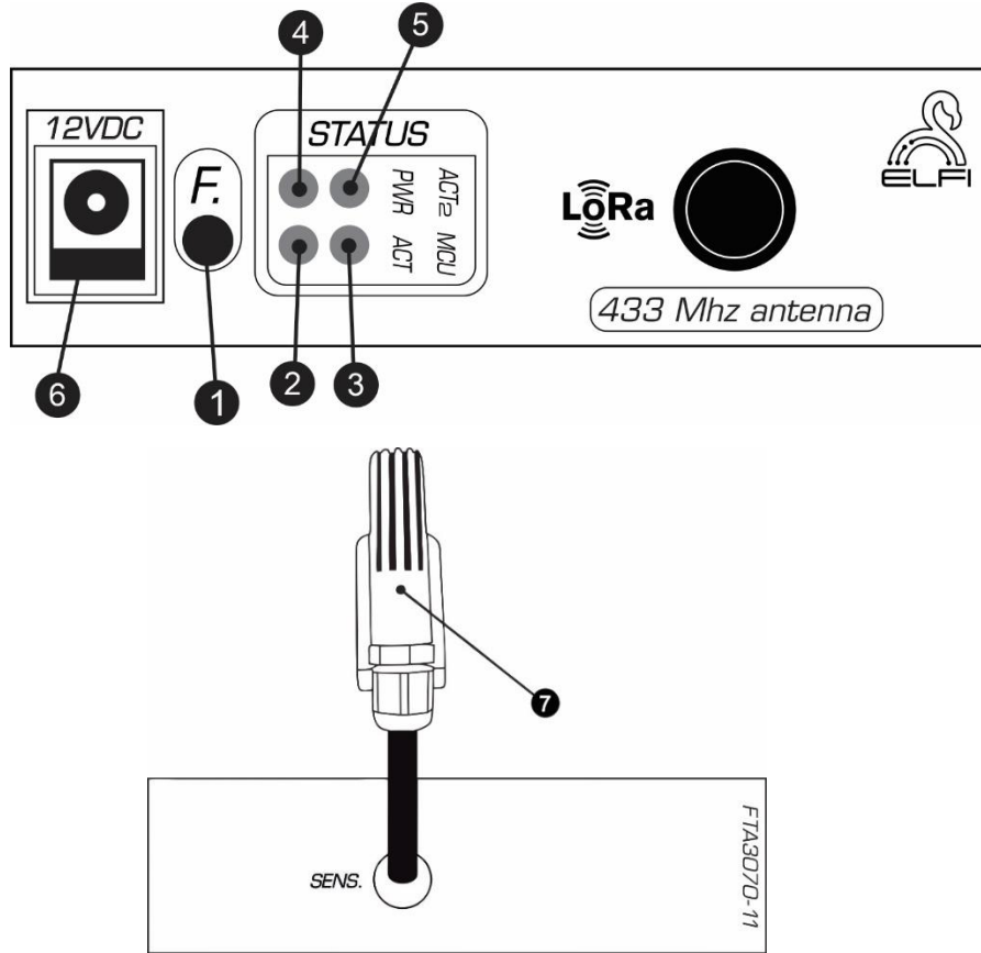
شکل ۲: نمای جانبی Node دما و رطوبت بی سیم
