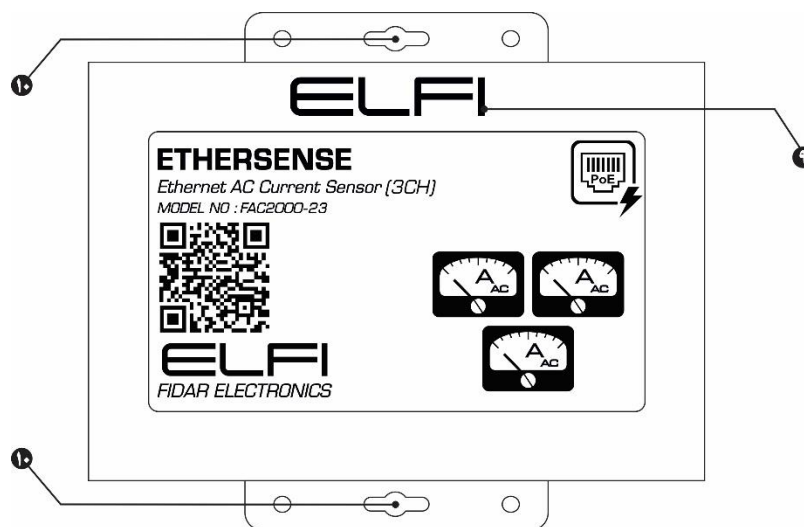
شکل ۳: نمای روبه روی سنسور جریان مستقیم
