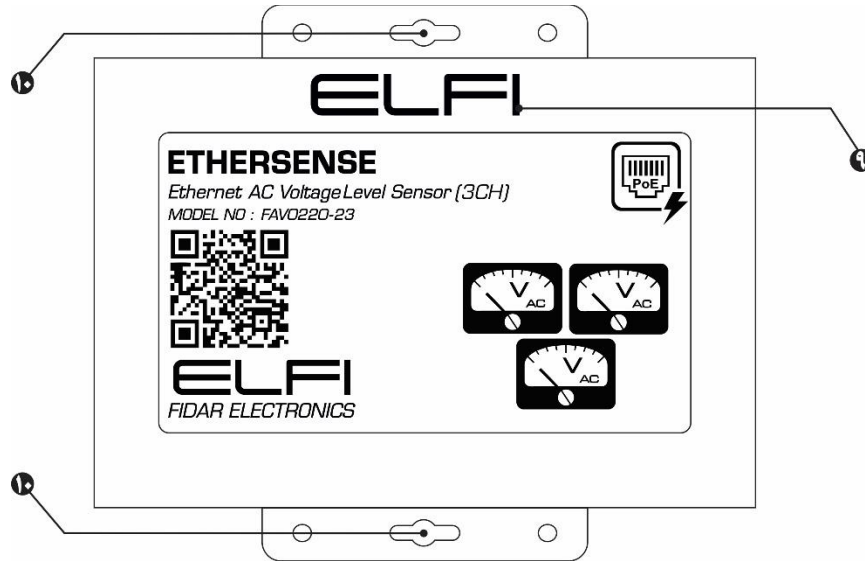
شکل ۳: نمای روبه روی سنسور سطح ولتاژ متناوب
