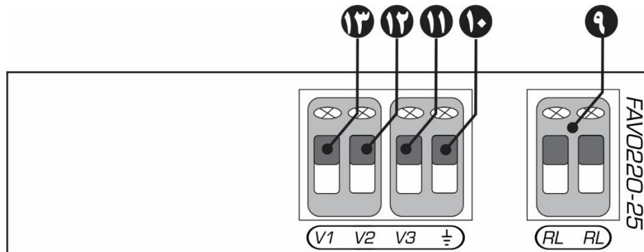
شکل ۴: نمای جانبی دتکتور ولتاژ متناوب سه کانال
