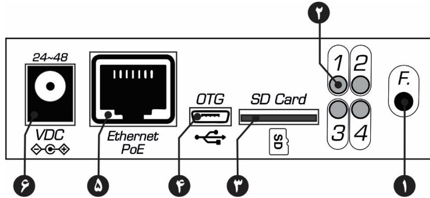
شکل ۲: نمای جانبی دتکتور ولتاژ متناوب سه کانال
