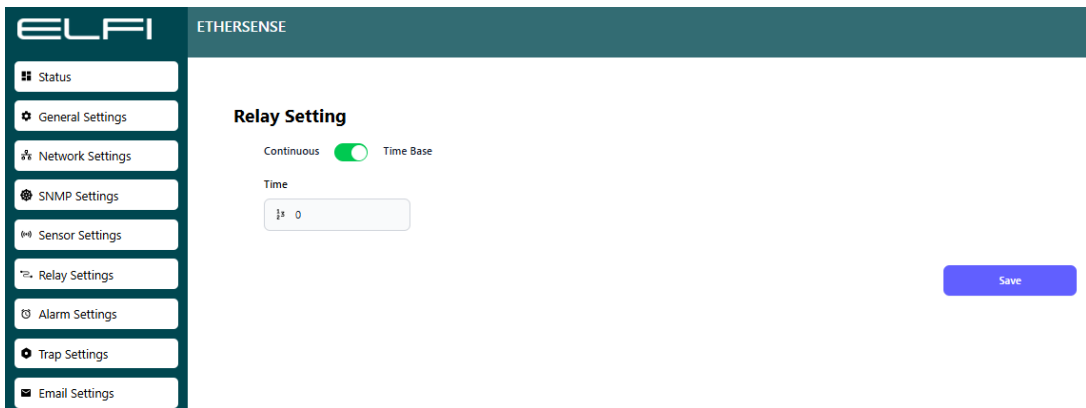
شکل ۱۱: منوی تنظیمات رله‌ی سنسور نشتی آب
